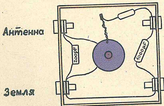
Чертеж 4. Монтажная схема радиоприемника
