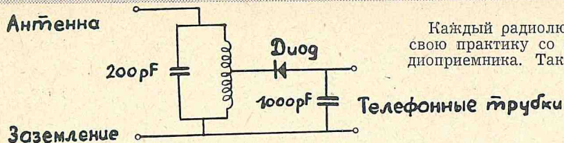
Чертеж 1. Принципиальная схема радиоприемника
