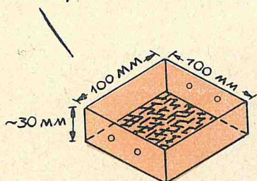
Чертеж 2. Приблизительные размеры коробки
