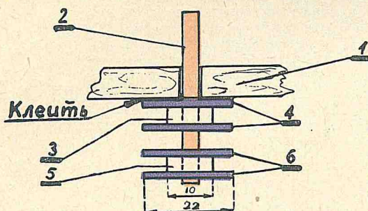
Чертеж 3. Изготовление и крепление сердечника дбуксекционной катушки радиоприемника
